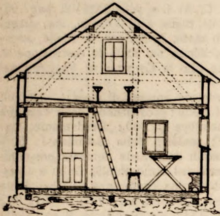
SEZIONE TRASVERSALE.
