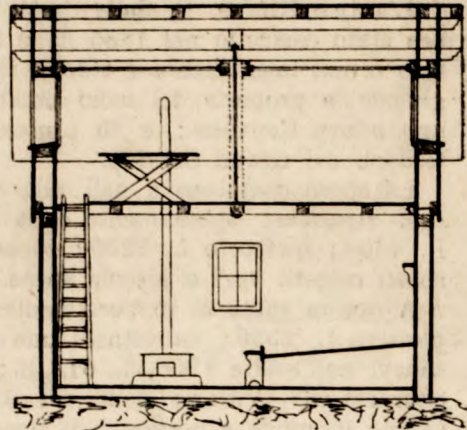
SEZIONE LONGITUDINALE.
